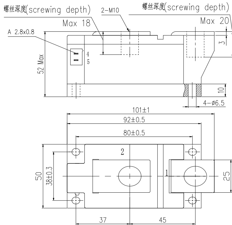
图7. 外形图
